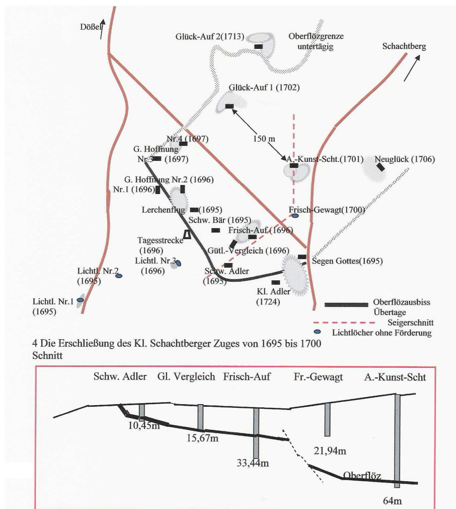
5. Schnitt durch den Kleinen Schachtberger Zug vom Schw. Adler zum A.-Kunst-Schacht
