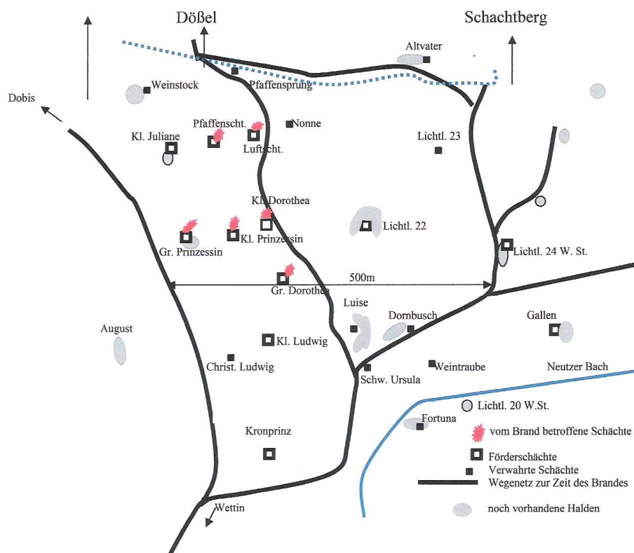
10 Situationsskizze der Schächte im Brandrevier 1739
